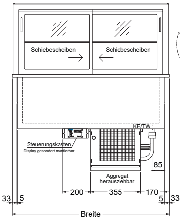
(Bedienseite)
