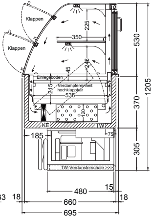
(Schnitt > rund)
